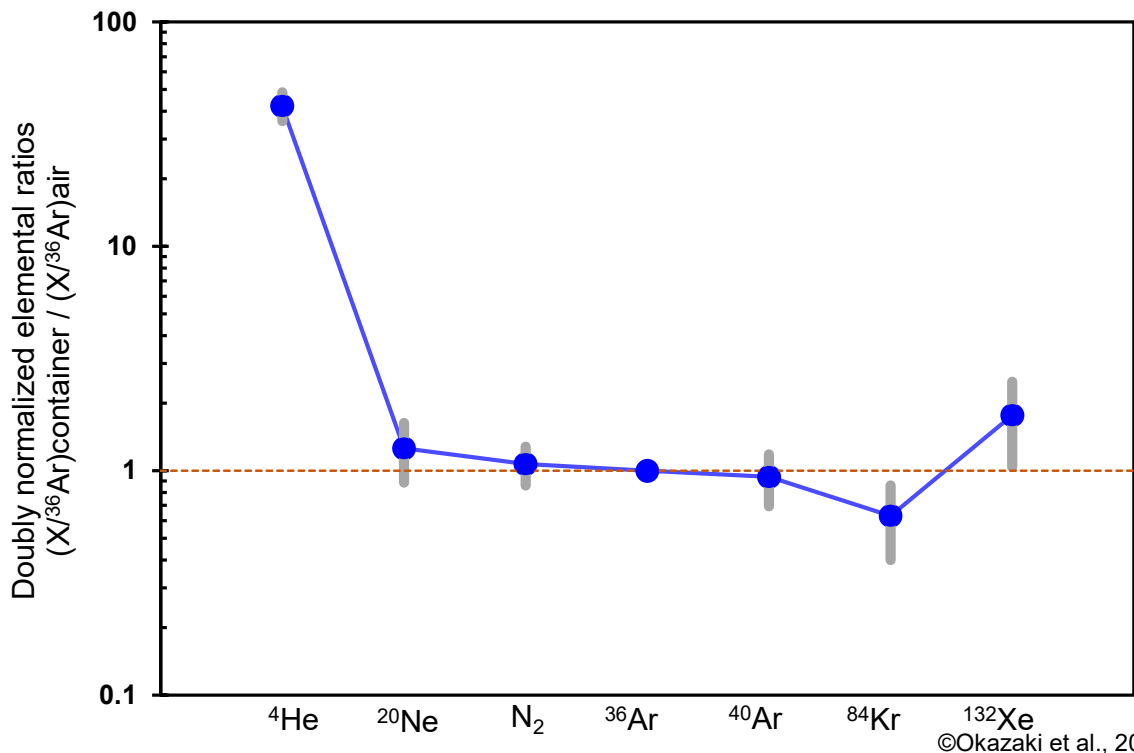
図 3: コンテナガスの元素存在度 (青実線)。測定誤差は灰色棒で示している。縦軸は 36 Ar と地球大気組成で規格化した存在度。横軸はガス種を示す。ヘリウムは地球大気 (オレンジ色点線) に比べてひと桁以上過剰である。
