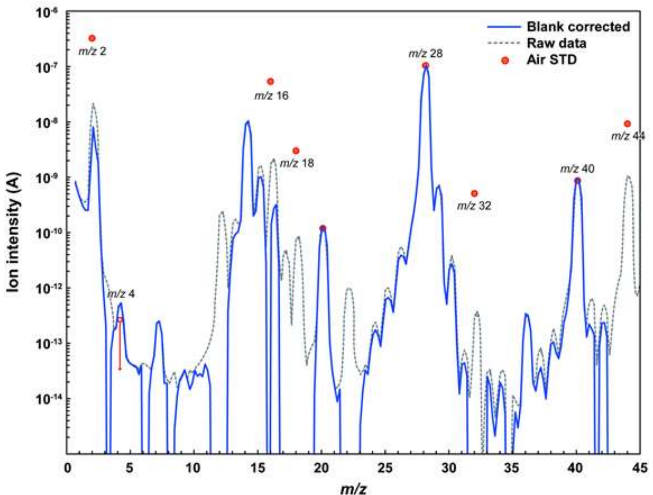
図 1: GAEA 搭載の質量分析装置によるコンテナガスの質量分析結果(青色実線)。横軸は質量(m)とイオン価数(z)の比(m/z)、縦軸は m/z に相当するイオンの質量分析装置での電気信号強度(任意スケール)。装置由来のガス(灰色点線)や地球大気標準ガス(赤丸)とくらべて m/z が4のガス(ヘリウム)が過剰に存在する。
