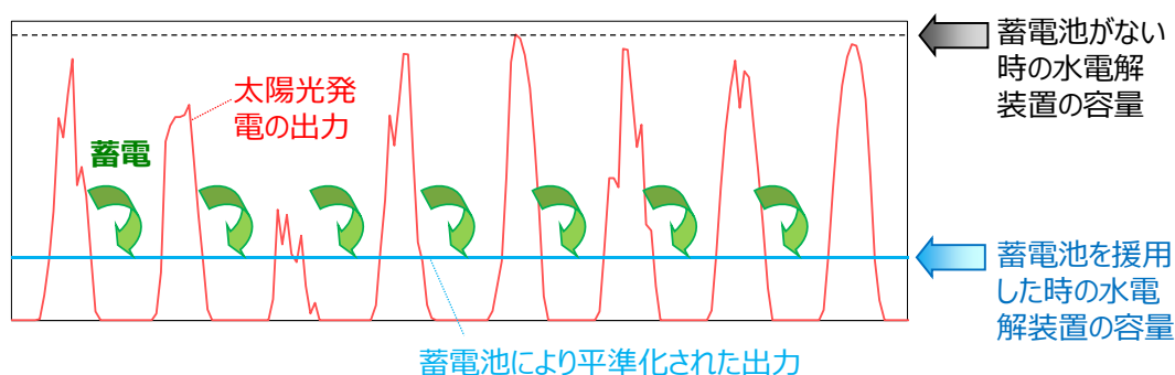
図 1 蓄電池の援用効果の模式図。日照により変動する太陽光発電の出力を蓄電池により平準化することで、水電解装置の設備容量を抑えるとともに稼働率を高めることができる。
