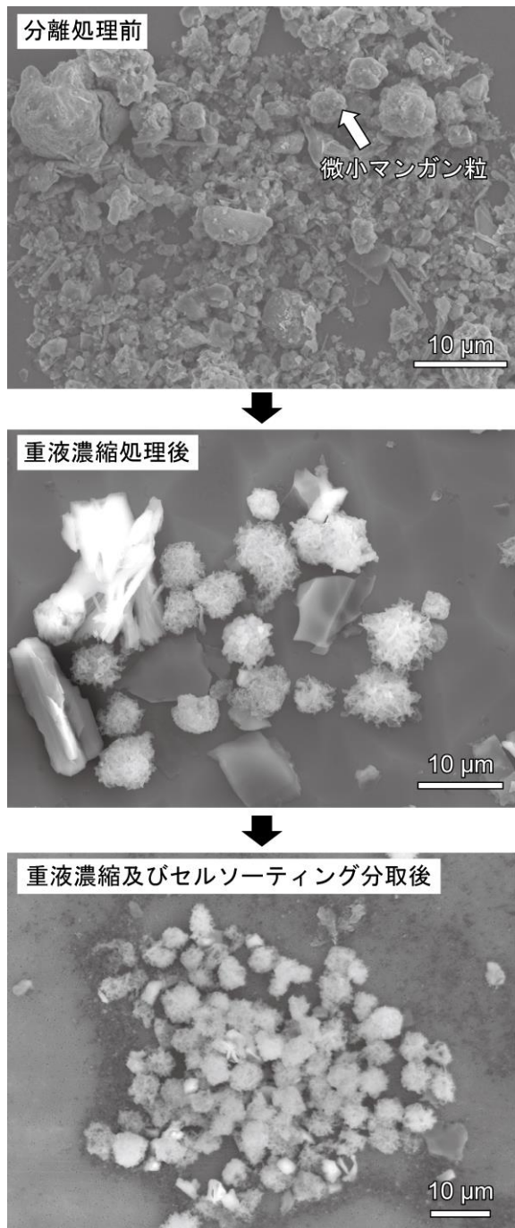
図5 微小マンガング粒の選別分離処理前後の走査電子顕微鏡写真。分離処理前（上）、重液処理後（中）、重液処理およびセルソーターによる分取後（下）。
