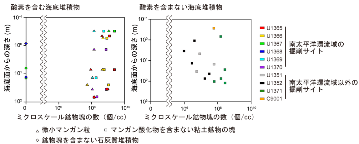
図3 海底堆積物試料 1 cc に含まれるミクロスケール鉱物塊の数の深度プロファイル。
