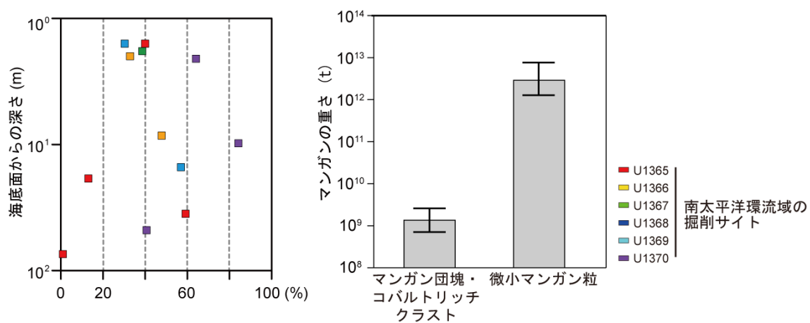
図4 南太平洋環流域の遠洋性粘土中に含まれる全マンガングに対し、微小マンガング粒に由来するマンガング割合の深度分布 (左) と、既知の海底金属酸化物・微小マンガング粒に含まれるマンガング量の比較 (右)。
