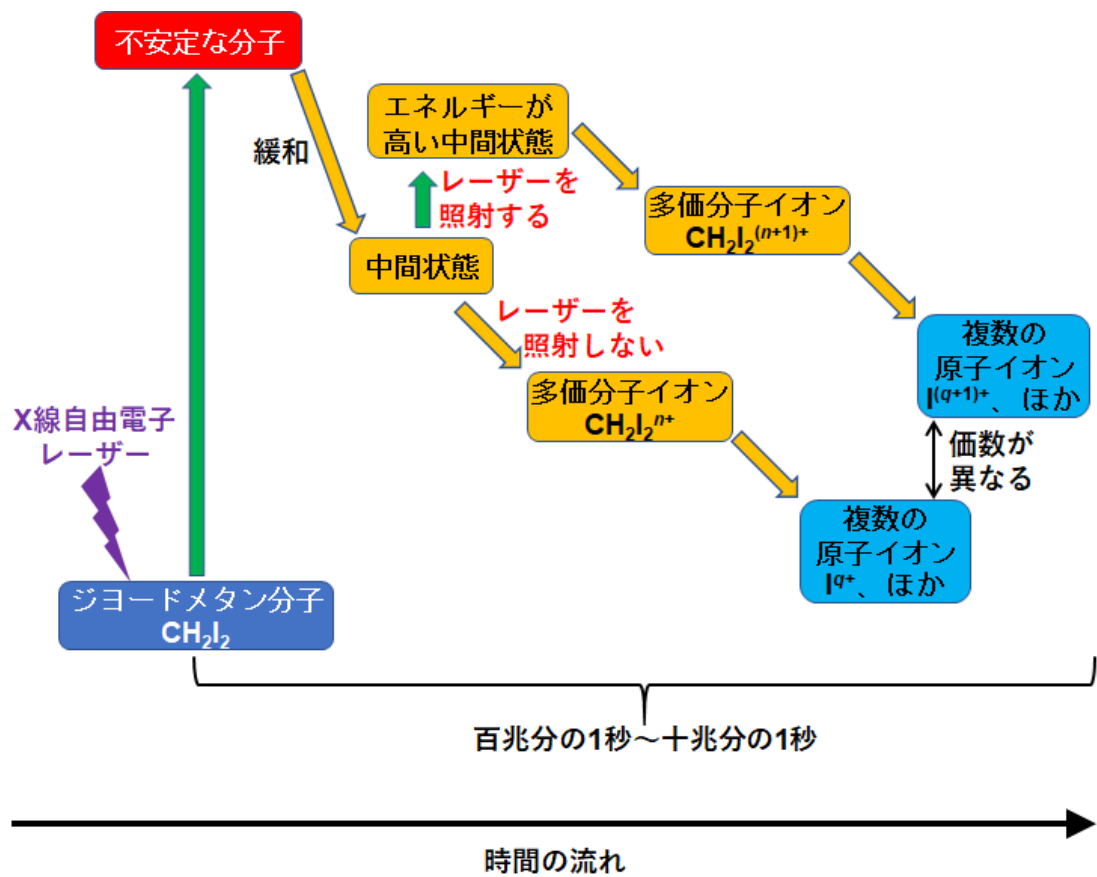
図 1. X 線照射によって起こる一連の過程の模式図
