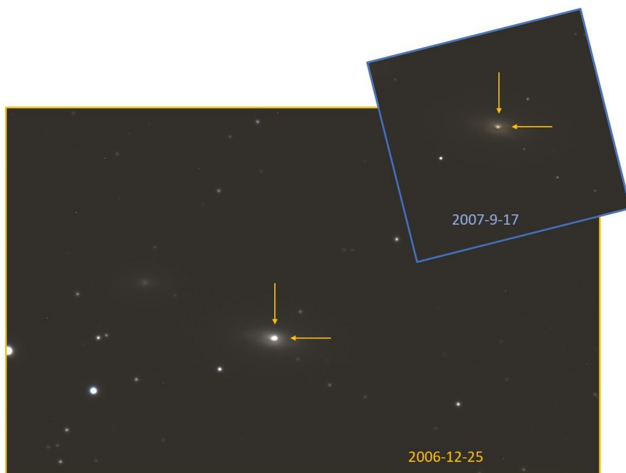
図 1 : 超高輝度超新星 SN2006gy のすばる望遠鏡 FOCAS による画像。発見から約 100 日後 (最大光度時) の 2006 年 12 月 25 日には SN2006gy の発生した銀河よりも明るく輝いているが、爆発後約 400 日後 (最大光度から約 300 日後) の 2007 年 9 月 17 日は非常に暗くなり、銀河そのものの明るさにほぼ埋もれてしまっている (© Koji Kawabata)。
