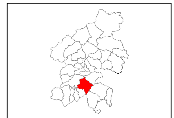
平成30年7月豪雨の土石流分布図と被災写真(板城小学校区)
