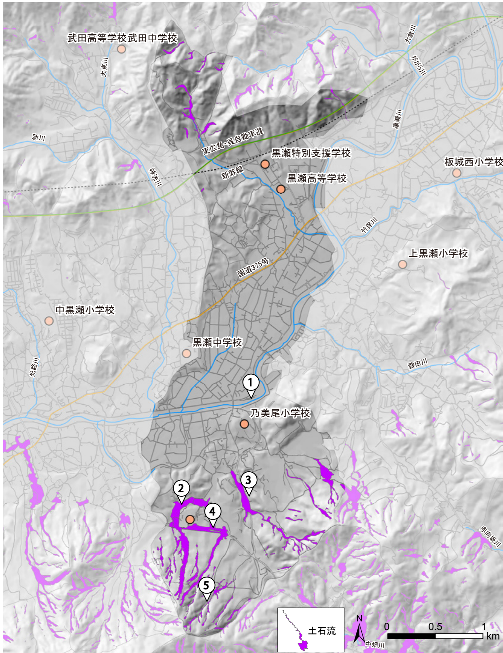
平成30年7月豪雨の土石流分布図と被災写真(乃美尾小学校区)
