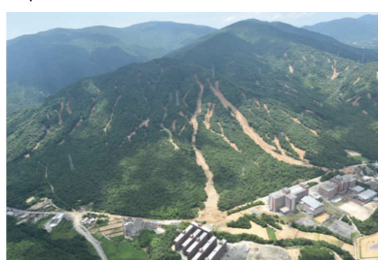
③ 前平山の土石流
