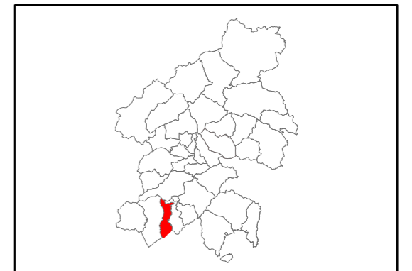
平成30年7月豪雨の土石流分布図と被災写真(乃美尾小学校区)
