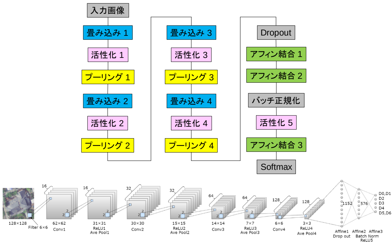
図 2 本研究で使⽤した畳み込みニューラルネットワークの構成
