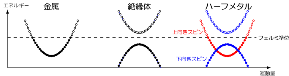
図3 金属/絶縁体/ハーフメタル強磁性体の典型的なバンド構造。 ●が電子を表し、○は電子の埋まっていない状態を表す。
