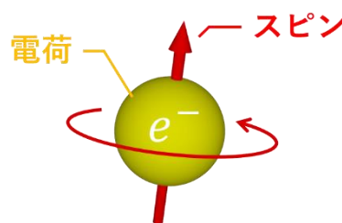
図2 電子スピンの概念図
