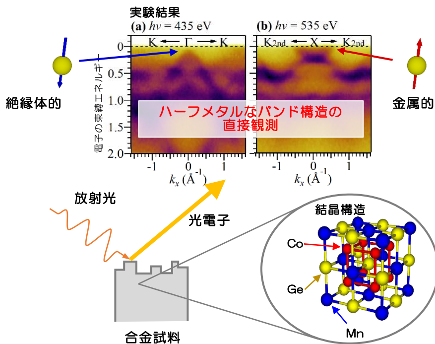
図 1 Co 2 MnGe の 3 次元な結晶構造（右下）に起因するでこぼこした試料表面のうち、限られた平坦面を絞られた放射光で狙い撃ちすることで（左下）、計算結果によってよく再現されるハーフメタルなバンド構造が観測された。（上）
