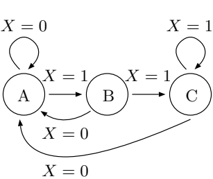
Figure 1: State machine 図 1 : ステートマシン
