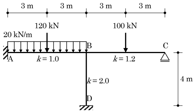
Fig. 1 Rigid frame
