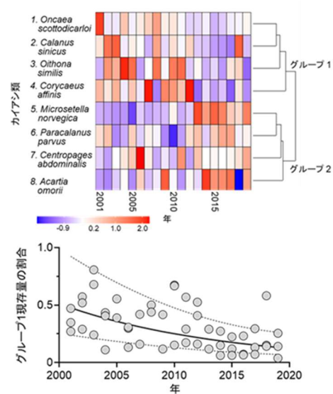
図2. 動物プランクトン(カイアシ類)8種の現存量の経年変化(上: 2001~2019年5~7月)およびカイアシ類全現存量に占めるグループ1現存量の割合の経年変化(下).
