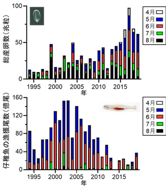
図3. 燧灘カタクチイワシの総産卵数(上)と仔稚魚の漁獲尾数(下)の経年変化(1994~2019年4~8月)。 上図: 産卵数は各月ともに最近年(2010年以降)に増加していましたが; 下図: 漁獲された仔稚魚(加入魚)は主に5月と6月に生まれていました; しかし、2000年代中盤から漁獲尾数が減少し、2010年以降、低位で推移していました
