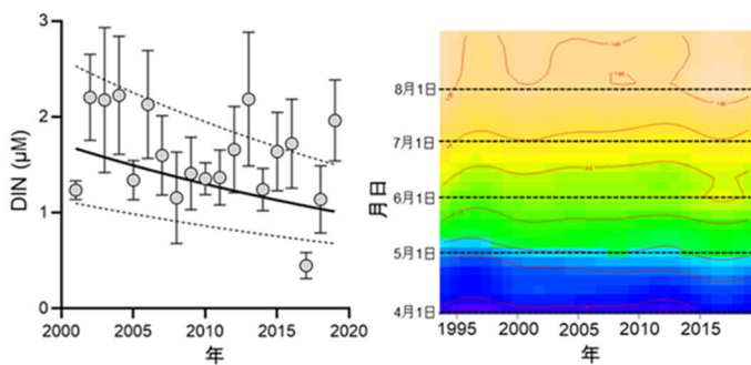
補足図1. 燧灘における溶存態無機窒素(DIN, 左; 2001~2019年4~7月)と水温(右; 1994~2019年4~8月)の経年変化。 左図: DINは経年的に減少していましたが; 右図: 5月の水温は経年的に高くなり、2015年以降では6月の水温も上昇していることが判りました(低: 青→緑→赤黄: 高)
