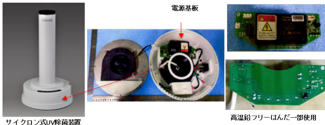
図3. コロナ殺菌クリーナ電源基板の一部に Bi 系高温鉛フリーはんだ実装搭載
