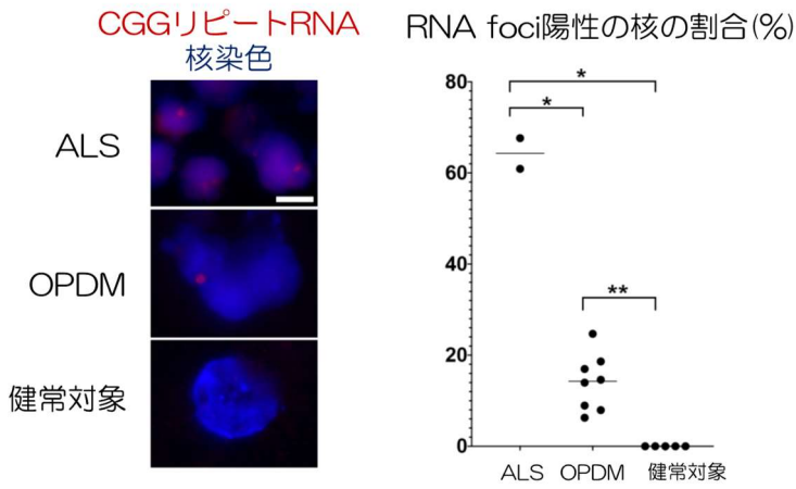
図 1. iPS 細胞由来運動神経の RNA foci
