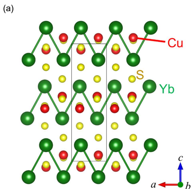
図 2: (a) \text{YbCuS}_2 の結晶構造。Yb 原子がジグザグ鎖を組む。(b) \text{YbCuS}_2 における核スピン-格子緩和率 1/T_1 の温度依存性。反強磁性で通常の磁性半導体では説明できない金属的な振舞いを見せる。
