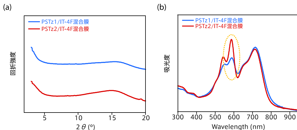
図3. (a) 開発したポリマーとIT-4F 混合薄膜のX線回折測定の結果。15° 付近の回折ピークが幅広で弱いことからアモルファスであることが分かる。(b) 開発したポリマーとIT-4F 混合薄膜の吸収スペクトル。PSTz2 では580nm 付近のピーク強度が顕著に大きく(黄色ハイライト部分)、ポリマー主鎖の平面性が高いことを示している。
