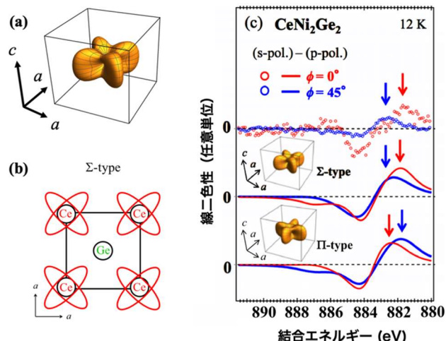
図1希土類超伝導体 \text{CeNi}_2\text{Ge}_2 の Ce 4f 電荷分布(a)と結晶 c 軸方向から見た Ce 4f 電子の軌道方向(b)、および硬 X 線光電子線二色性スペクトル(c)
