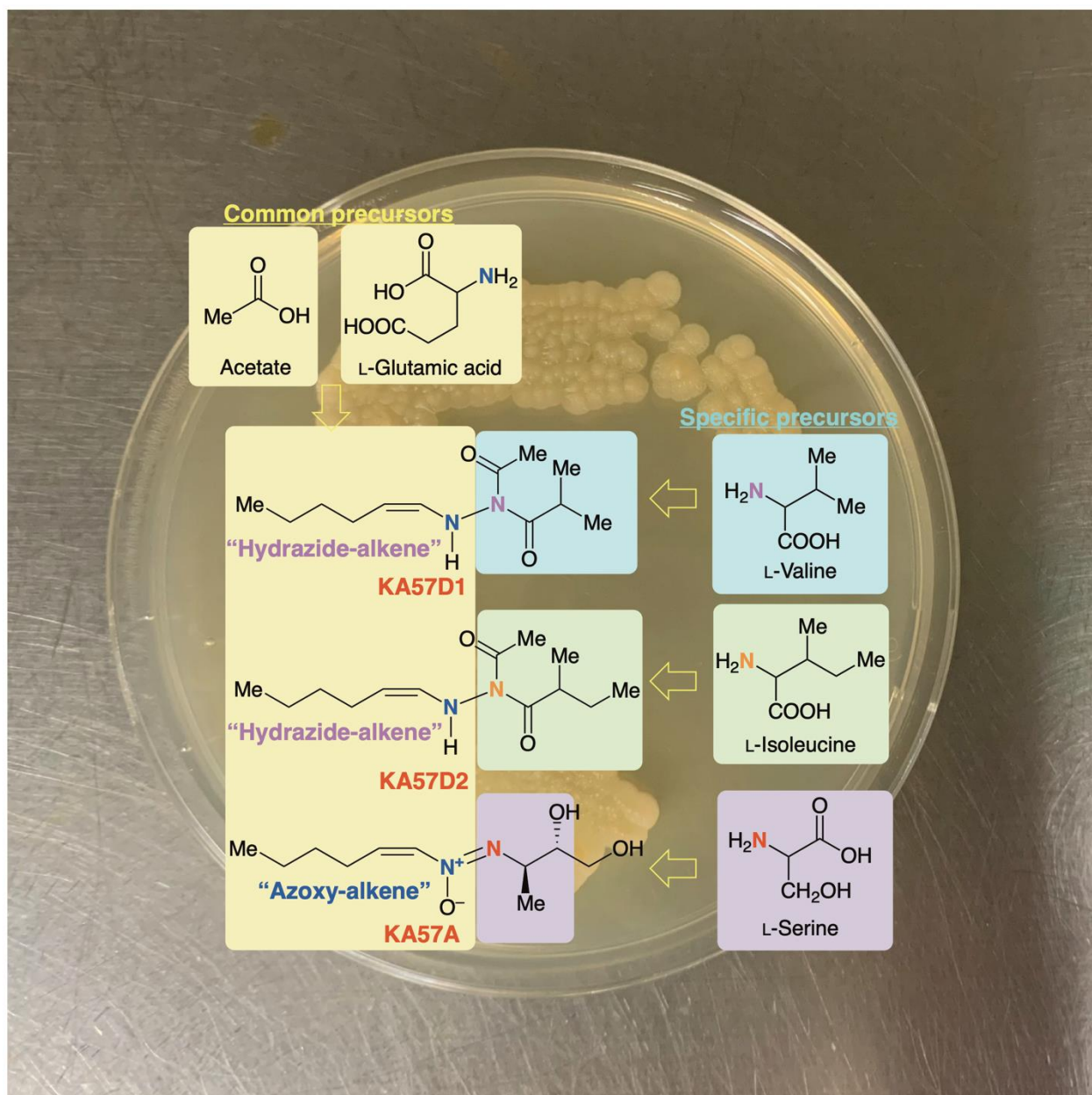
図 放線菌 Streptomyces rochei KA57 株の寒天上での生育およびアゾキシアルケン化合物 KA57A、ヒドラジドアルケン化合物 KA57D1、KA57D2 の生合成起源
