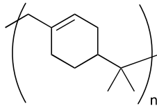
1,4-シクロヘキセニル構造
