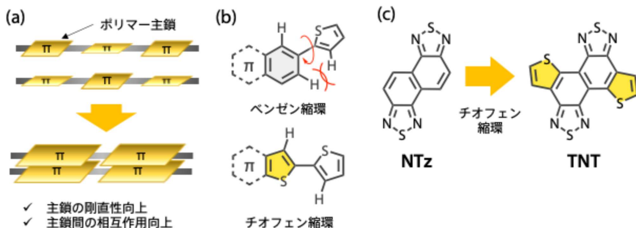
図 1. (a) ポリマー半導体の模式図。ビルディングユニット ( \pi 電子系骨格) の構造拡張により、ポリマー主鎖の剛直性や相互作用が向上する。(b) 構造末端にチオフェンを縮環することによる効果。例えば、6 員環であるベンゼンを縮環したときに比べると、5 員環であるチオフェンを縮環することで、立体障害が軽減され、ポリマー主鎖の共平面性が向上し、より剛直性や相互作用が向上する。(c) 広島大学の研究グループがこれまで用いていた縮環 \pi 電子系骨格「NTz」と本研究で開発したチオフェン縮環 \pi 電子系骨格「TNT」の化学構造。
