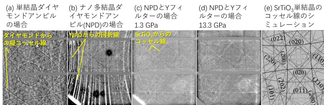
図2 DAC 中の \text{SrTiO}_3 単結晶試料から得られた高圧下ホログラム像。NPD アンビルと Y フィルターによって、高圧下でも \text{SrTiO}_3 試料の単結晶性に由来するコッセル線を含む明瞭なホログラム像が得られた。
