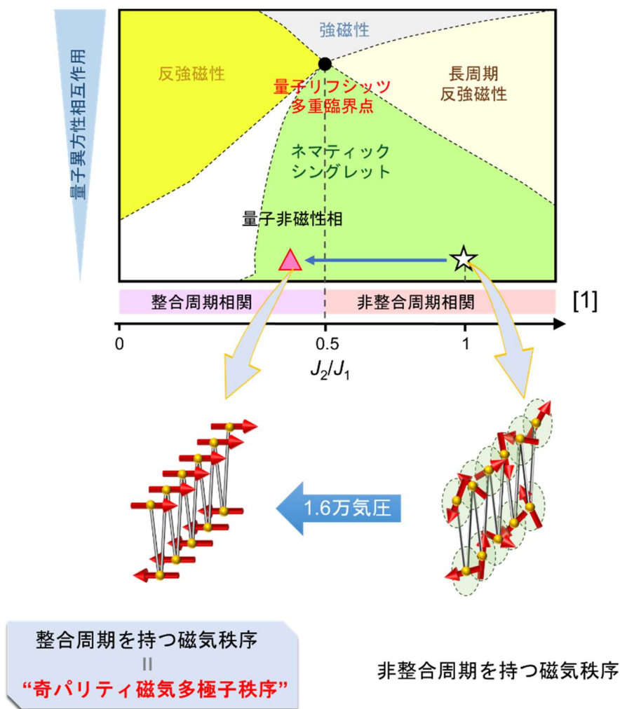
図 1: YbCuS 2 の圧力による状態変化と理論予測[1]との比較。1 気圧下で見られた非整合な螺旋磁気秩序が、1.6 万気圧下では整合周期を持つ別の磁気秩序に変化する。この高圧下の状態は「奇パリティ磁気多極子秩序状態」と呼ばれる特異な秩序状態である。赤矢印は Yb のスピン（角運動量）の向きを表す。
