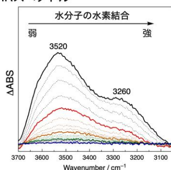
図 3：細孔界面から第二水和圏の水分子の IR および XES スペクトル
