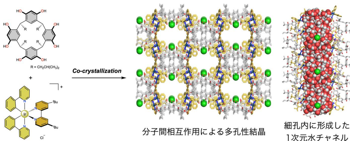
図 1: 環状有機ホストと錯塩からなる多孔性結晶の合成と 1 次元水チャンネルの形成. ナノ細孔を正面（中央図）および横から見た図（右図）。塩化物イオンを緑色球体で示している。
