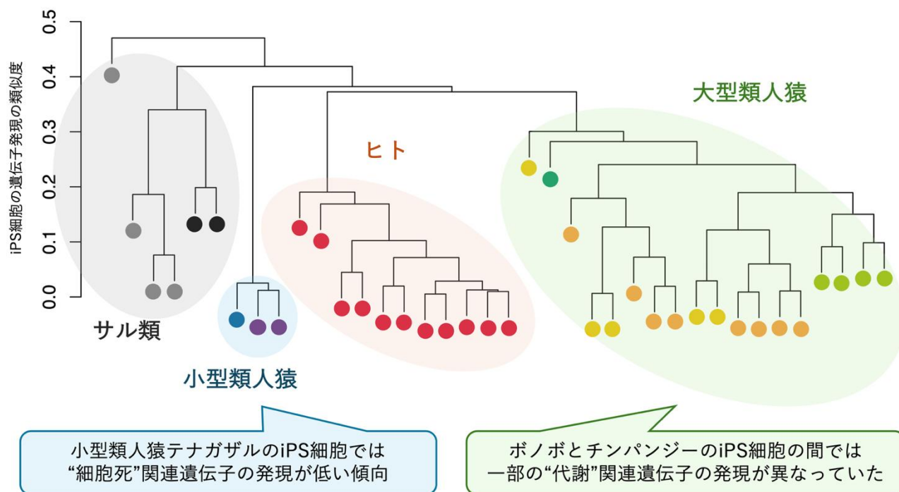
図 3. 類人猿の iPS 細胞から四肢骨格の起源である肢芽中胚葉細胞の分化誘導に成功
