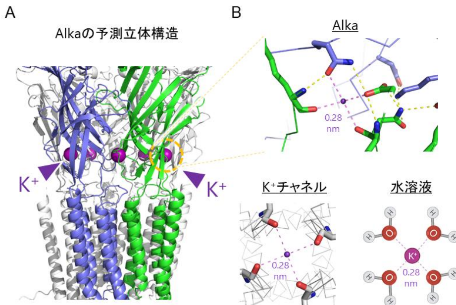
図 3 Alka が K^+ を認識する原子レベルでのメカニズム
