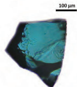
マントル遷移層上部の主要構成鉱物
