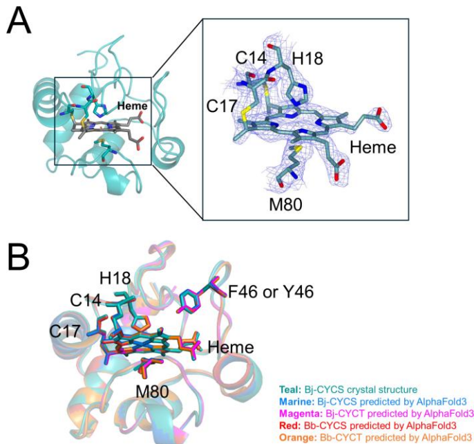
図 4 ヘムの近くに位置する 46 番目のアミノ酸
