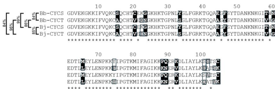
図2 カエル2種のアミノ酸配列と組織ごとの遺伝子発現
