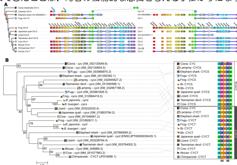
図1 2つの cyc 遺伝子の起源を示す遺伝子の並びと系統関係
