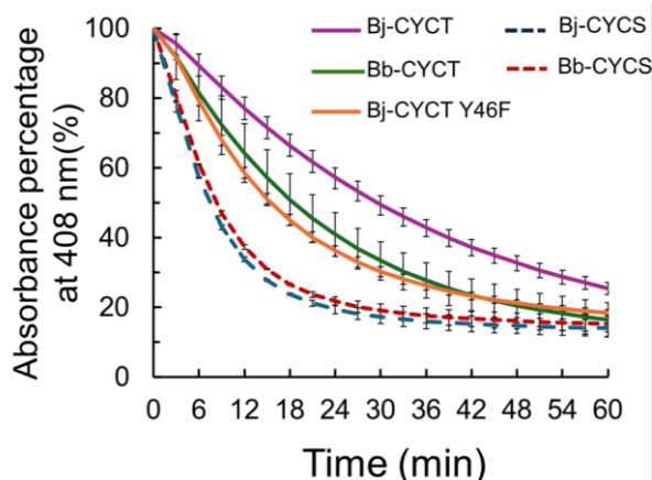
図3 精巣型シトクロムcの過酸化水素耐性
