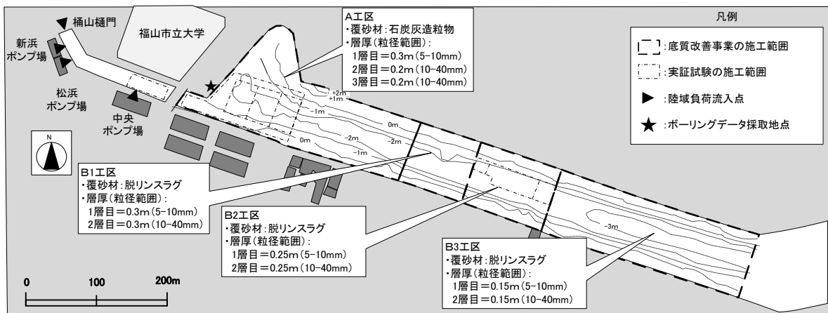
福山内港における底質改善の実施箇所と使用材料および施工層厚
