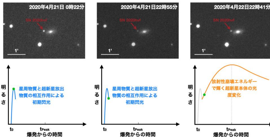
図 1. 上半分の三枚の画像は、Tomo-e202004aaelb (SN 2020hvf)の最初期の Tomo-e Gozen による観測画像（2020年4月20日から約一日おきの画像）。下は、同じ時刻における光度の進化の様子（時間に対して光度を示した、光度曲線）。緑の点は、上の超新星観測時と対応する光度の段階を示す。（Credit：Kavli IPMU/東京大学）
